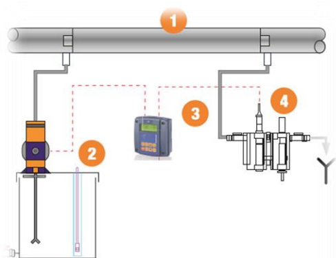
Linha água Sistema de dosagem/ prod. químico Controlador Compact Alojamento Sensor/ DGMA
