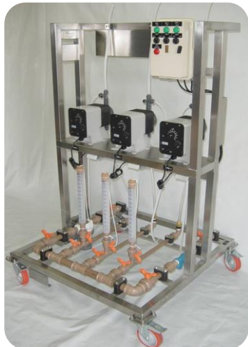
Skid 03 bombas dosadoras com provetas e estrutura inox .
